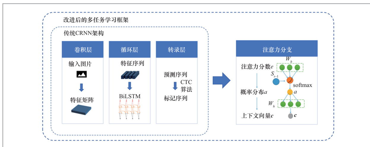
图5 引入注意力分支的多任务学习框架
