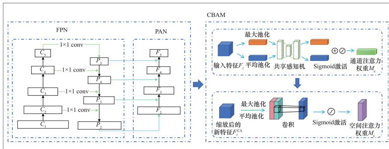
图4 引入多尺度空间注意力的检测模型架构
